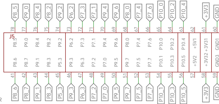
MSP432LAUNCHPAD_J5
