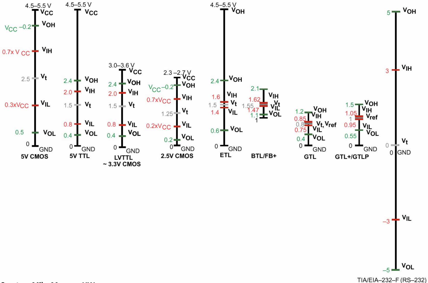
TIA/EIA-232-F (RS-232)
