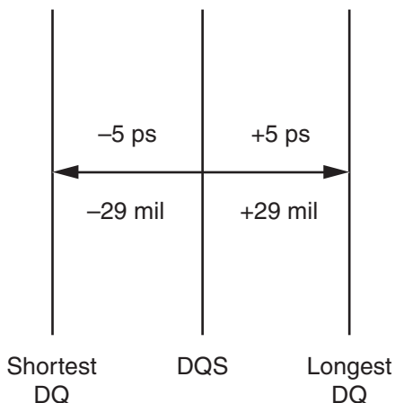
Figure 2-4: Skew Example for DQ to DQS
