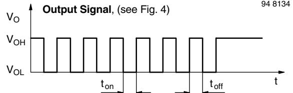
Fig. 3 - Output Function
